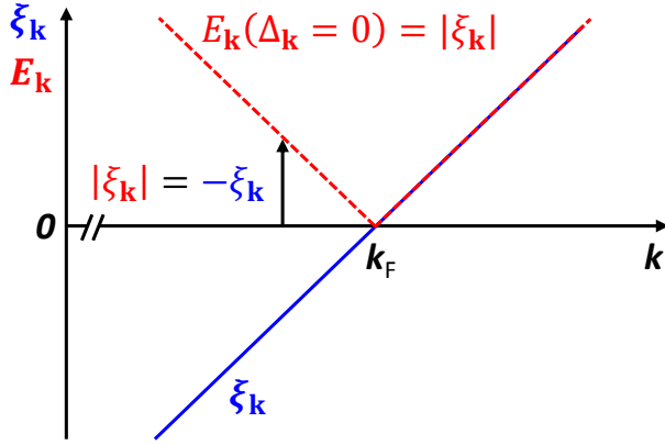
Figure 1: Zur Definition der Energien E_{\mathbf{k}}(\Delta_{\mathbf{k}} = 0) = \sqrt{\tilde{\zeta}_{\mathbf{k}}^2 + \Delta_{\mathbf{k}}^2} = |\tilde{\zeta}_{\mathbf{k}}| und \tilde{\zeta}_{\mathbf{k}} in der Nähe der Fermi-Wellenzahl k_{\text{F}} .
